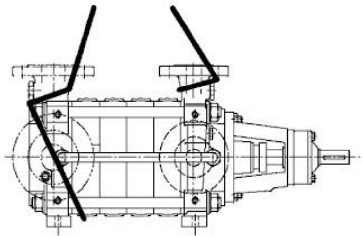
Рис. 1 Схема строповки насоса
