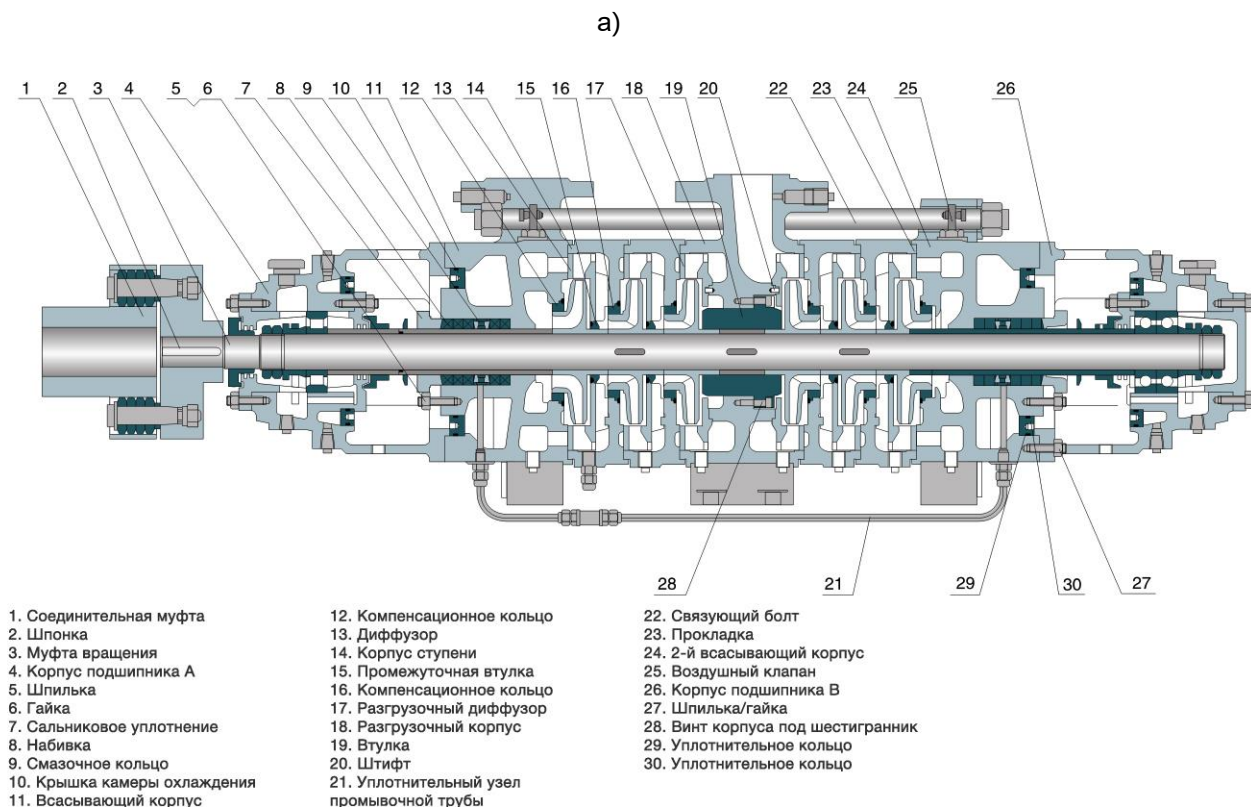
Рис. 11 Разрез насоса СМВ
